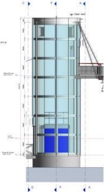
B Aanzicht lift west schaal 1:50
