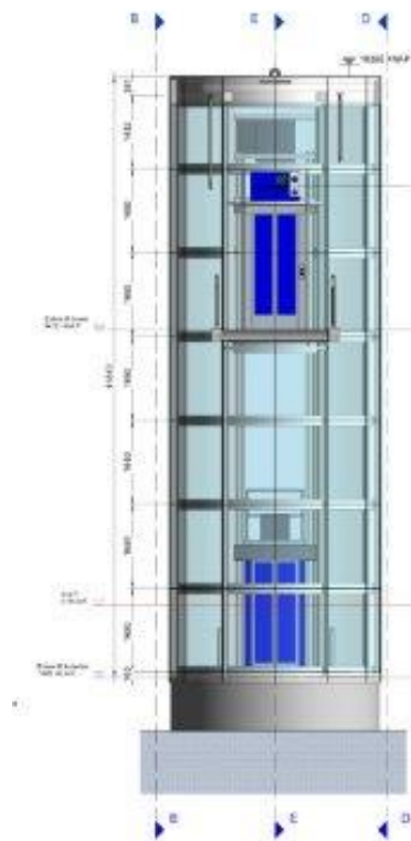
A Aanzicht lift zuid schaal 1:50
